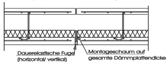
Syspro Part Thermowand Fugendetail
